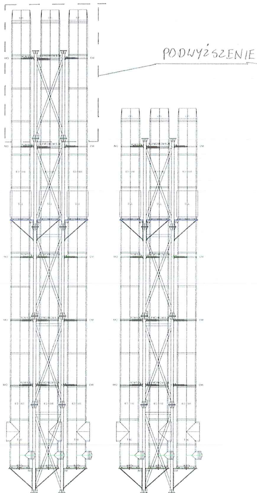
STAN PROJEKTOWANY — ISTNIEJĄCY STAN Szkic podwyższenia konstrukcji kominów
